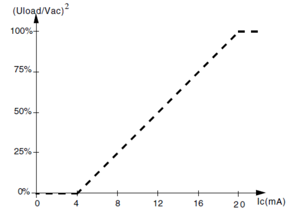
Fig.3 Caractéristique de transfert, linéarisé en U 2
