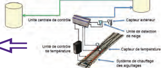
Système de contrôle principal
